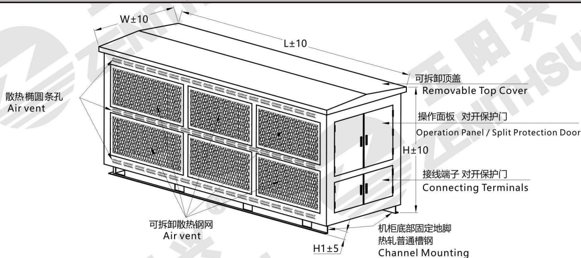
智能负载箱尺寸表(单位:mm) / Dimensions (mm)
