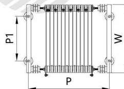
图三 (俯视图)
