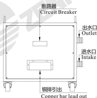
图一 (主视图)
