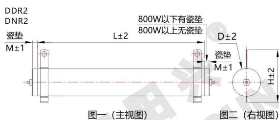
图一 (主视图)
