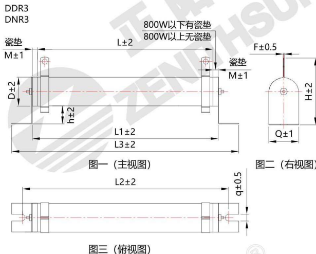
图三 (俯视图)
