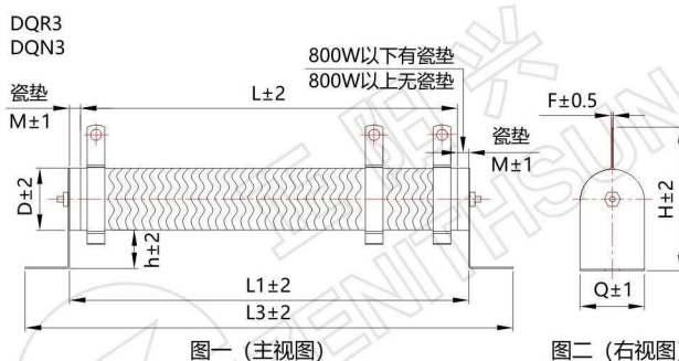
图一 (主视图)
